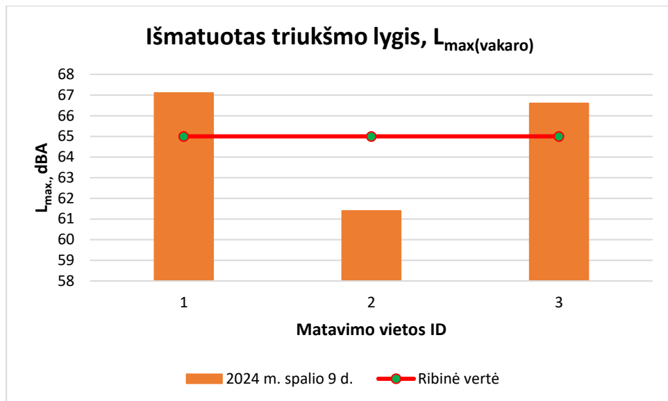
42 pav. Maksimalaus triukšmo pasiskirstymas matavimo vietose vakaro metu (19 – 22 val.). Ribinis dydis 65 dBA
