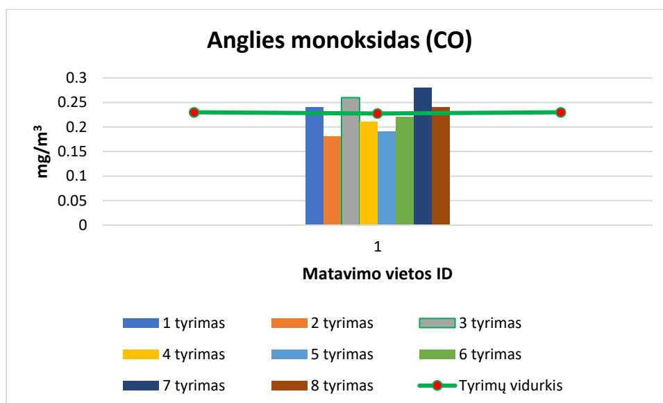
13 pav. Anglies monoksido koncentracijų pasiskirstymai Alytaus rajone pagal nustatytos matavimo vietos ID. (Ribinė vertė 10 mg/m 3 grafike neatvaizduojama, nes gautos CO koncentracijų vertės ženkliai mažesnės)
