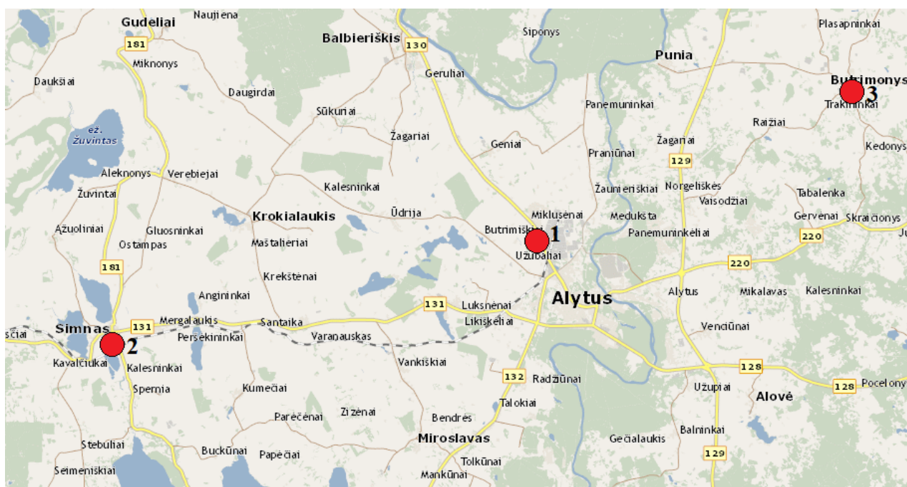
14 pav. Aplinkos triukšmo monitoringo tinklas Alytaus rajono savivaldybėje
