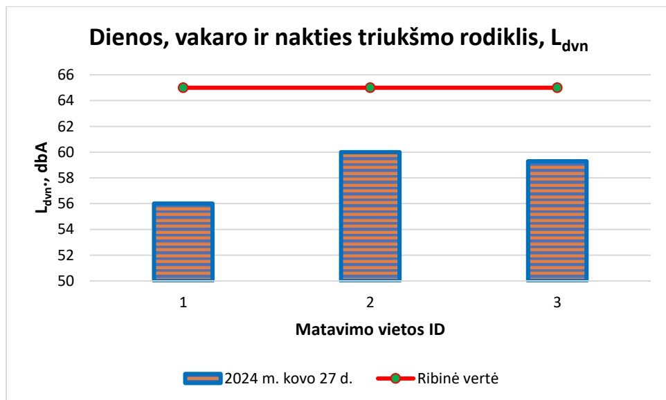
22 pav. Dienos, vakaro ir nakties triukšmo rodiklio ( L_{\text{dvn}} ) pasiskirstymas matavimo vietose. Ribinis dydis 65 dBA
