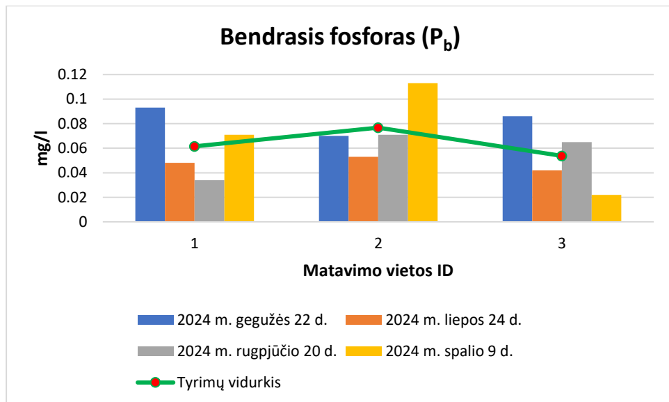
52 pav. P bendrojo koncentracijų pasiskirstymas vandens telkiniuose Alytaus rajone, nustatytose matavimų vietose. (Ribinė vertė 1,6 mg/l grafike neatvaizduojama, nes gautos P_b koncentracijų vertės ženkliai mažesnės)
