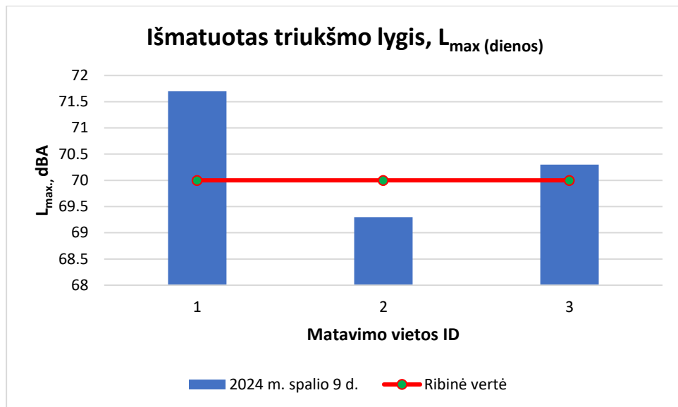
40 pav. Maksimalaus triukšmo lygio pasiskirstymas matavimo vietose dienos metu (7 – 19 val.). Ribinis dydis 70 dBA
